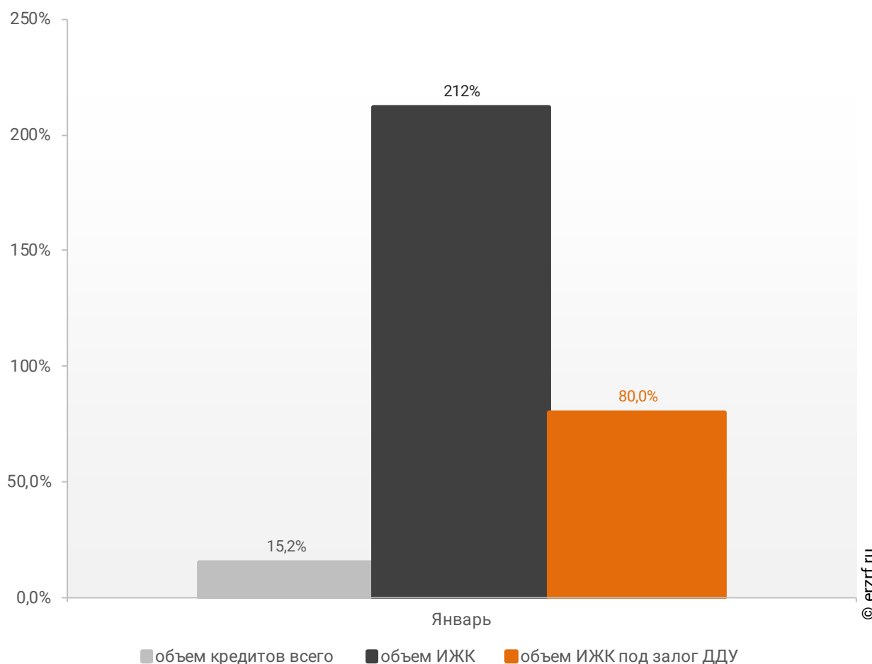
Динамика прироста объема кредитования по месяцам 2021 года по сравнению с аналогичными месяцами 2020 года в Чеченской Республике (по видам кредитов)
