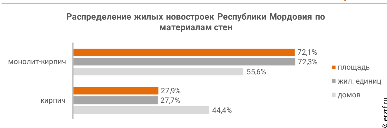
Гистограмма 5
